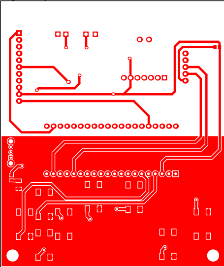
Top Layer (Scale 1:1.39198218262806)
