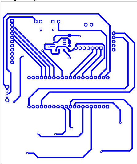
Bottom Layer (Scale 1:1.42714428428714)
