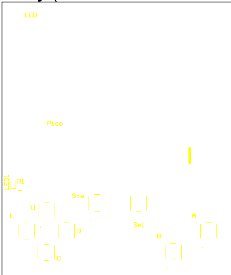
Top Overlay (Scale 1:1.39742873113471)
